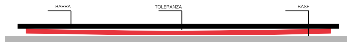
Configurazione per la corretta misurazione dell'imbarcamento
