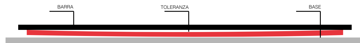
Configurazione per la corretta misurazione dell'imbarcamento
